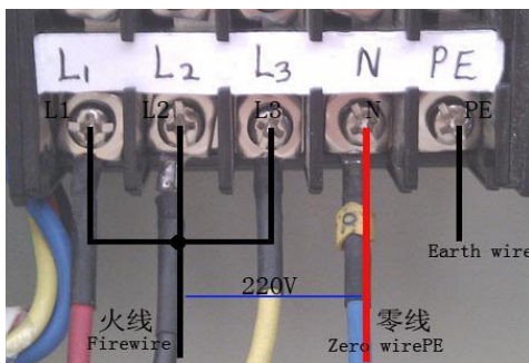
(220V 接线图)
