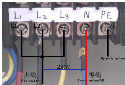
(220V 接线图)
