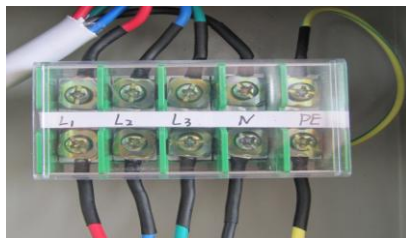
(380V 接线图)
